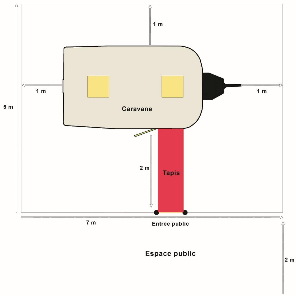
Plan d'implantation
